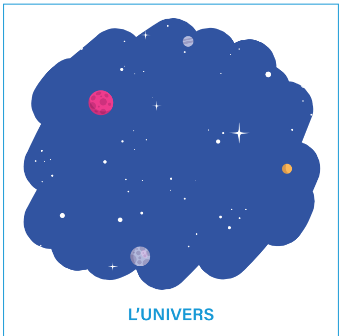
LE SYSTÈME SOLAIRE
